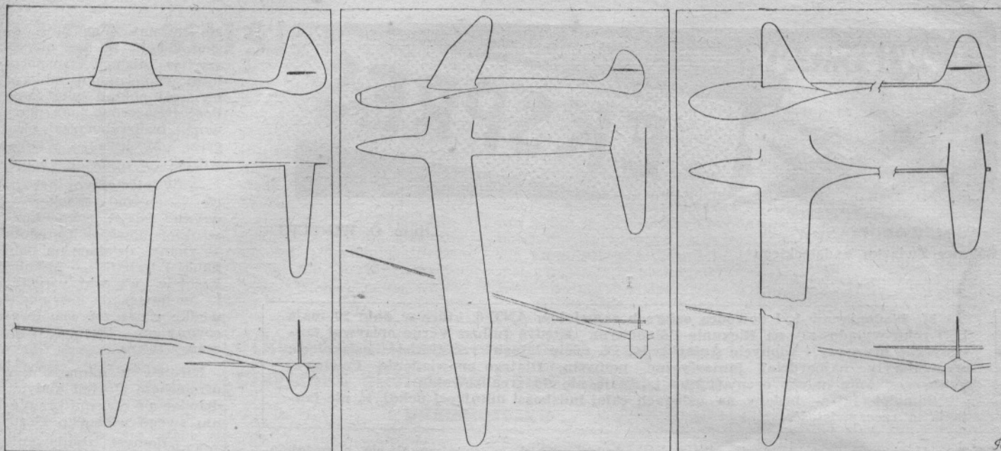
Szybowiec II P. Motekajtisa
